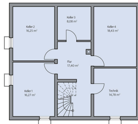
Haus Ernst Grundriss
