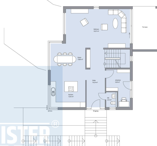
Haus Messerschmidt Grundriss
